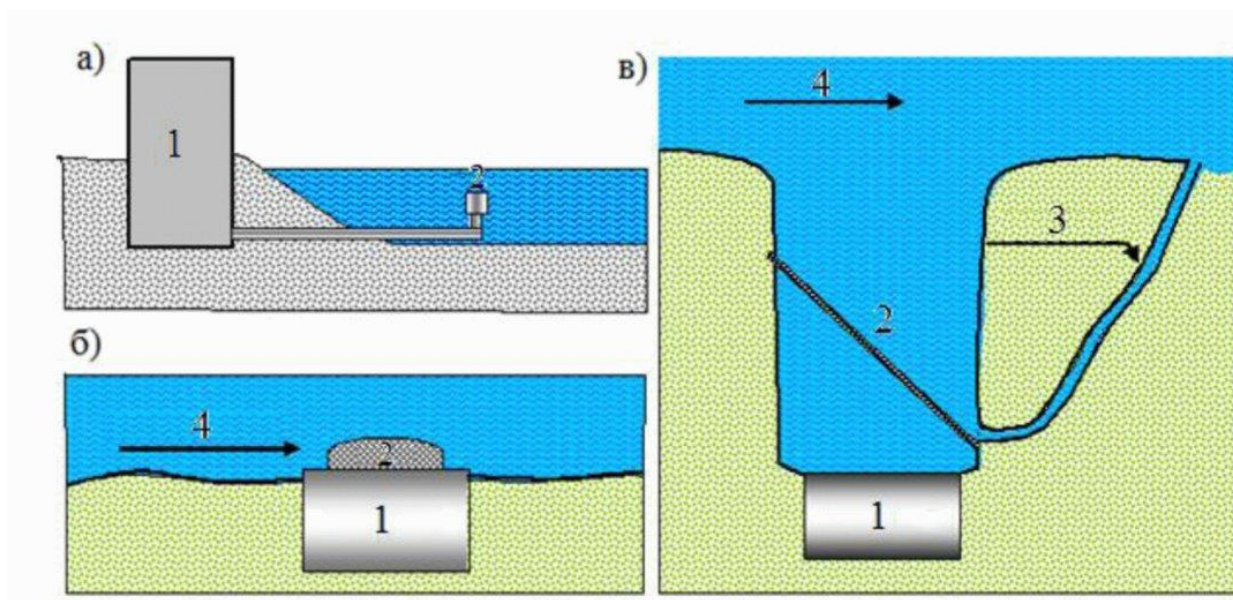
а - русловой оголовок; б - рыбозащитное сооружение, размещенное в водоприемной части; в - отдельно стоящее рыбозащитное сооружение; 1 - гидротехническое сооружение и (или) устройство забора воды; 2 - рыбозащитное сооружение; 3 - рыбоотвод; 4 - транзитный поток
