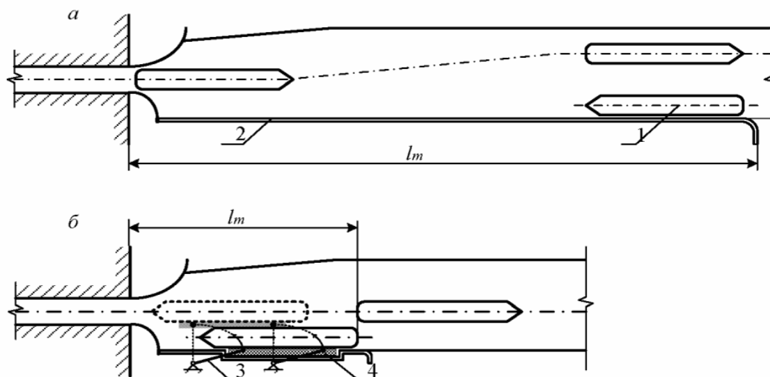
a - традиционная; б - с использованием причально-наводочного устройства 1 - судно; 2 - причальная линия; 3 - направляющие штанги; 4 - понтон; l_m - длина причальной линии
